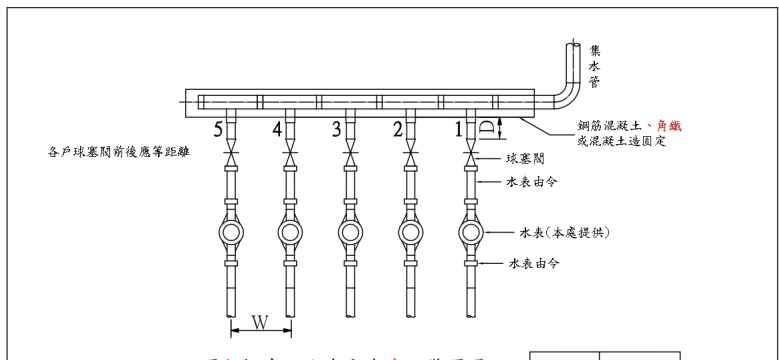
圖4-1 中、小表分表表位裝置圖
