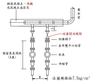
圖4-2 大表分表表位裝置圖
