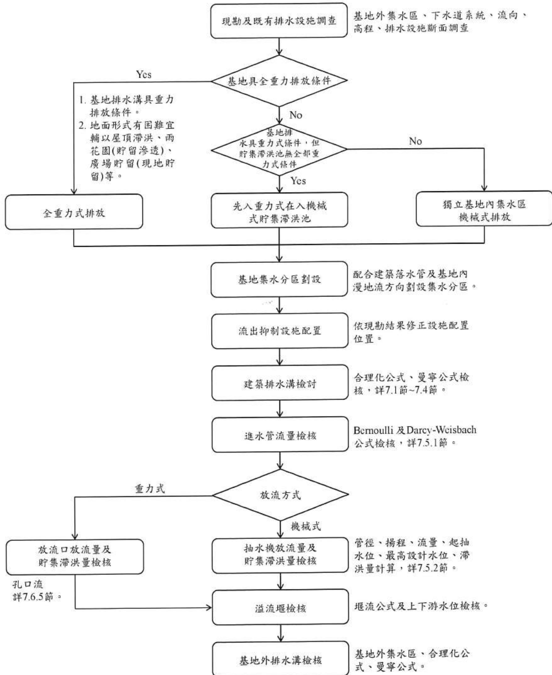
圖 7-2 設計流程圖
