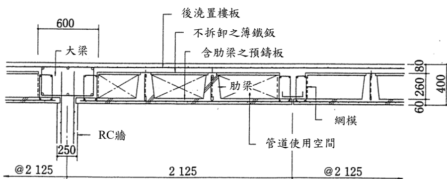
圖 R7.28 含肋梁之預鑄板構成之中空樓板例 [7.5]
