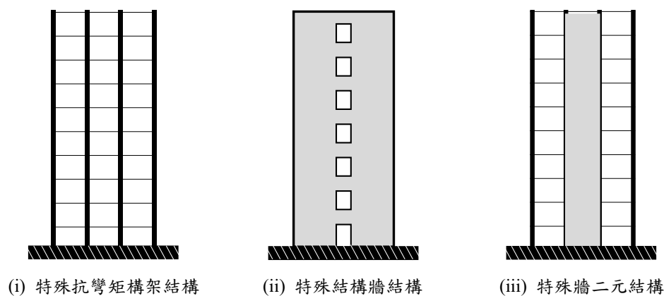
圖 R3.1 結構型式示意
