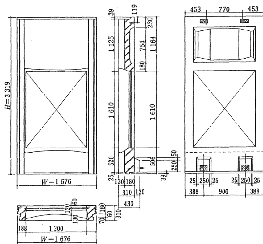
圖 R7.33 加肋帷幕牆圖例(單位：mm) [7.5]
