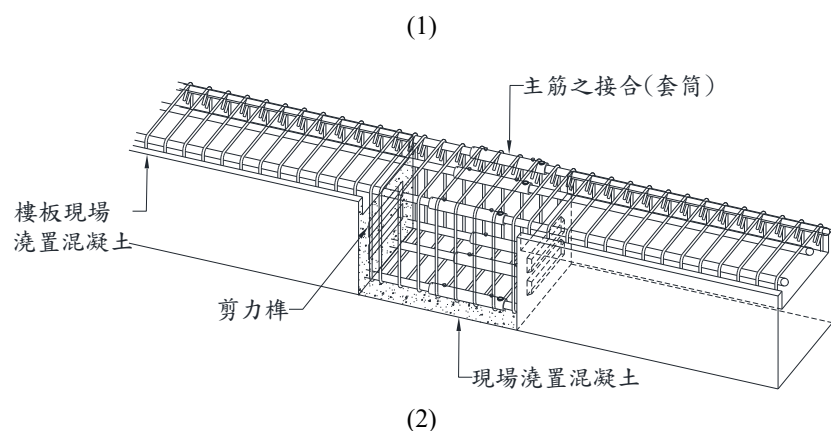
圖 R7.11 梁與梁接合圖例 [7.5]
