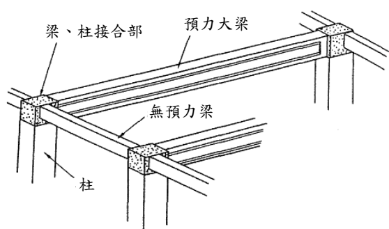
圖 R7.16 構架方式之構成構材例 [7.5]
