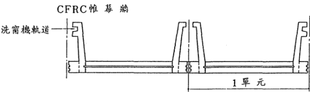
圖 R7.39 CFRC 帷幕牆圖例 [7.5]
