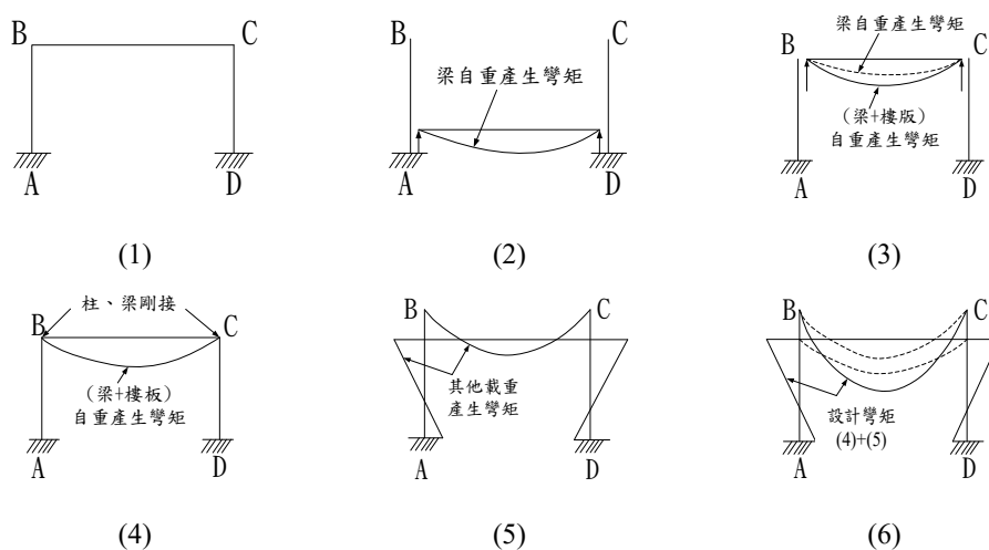
圖 R7.17 各施工階段應力 [7.5]
