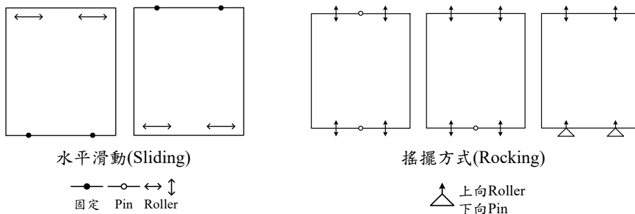
圖 R7.35 板式帷幕牆之接合設計原理 [7.5]
