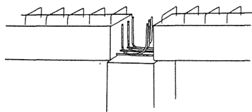
圖 R7.11 梁與梁接合圖例 [7.5]
