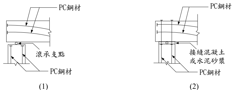
圖 R7.19 不產生二次應力之接合法例 [7.5]
