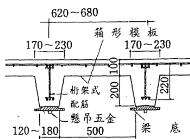
圖 R7.23 加肋樓板標準斷面例(單位：mm) [7.5]
