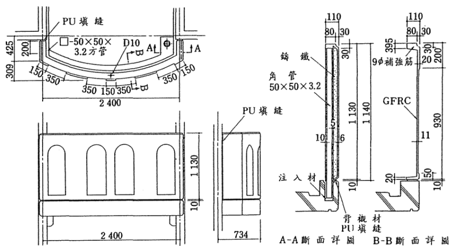
圖 R7.38 陽台扶手圖例(單位：mm) [7.5]
