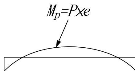
圖 R7.18 預力彎矩圖 [7.5]
