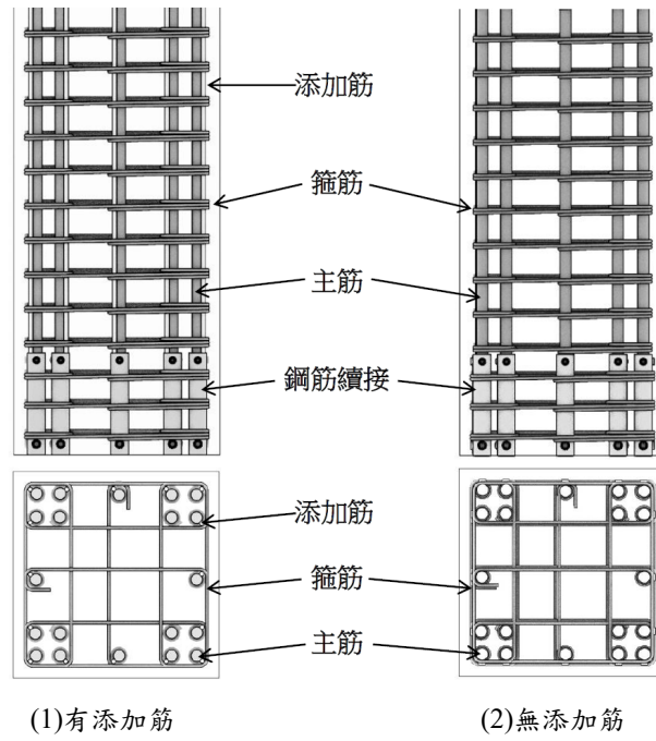
圖 R7.13 套筒方式接續之配筋圖例
