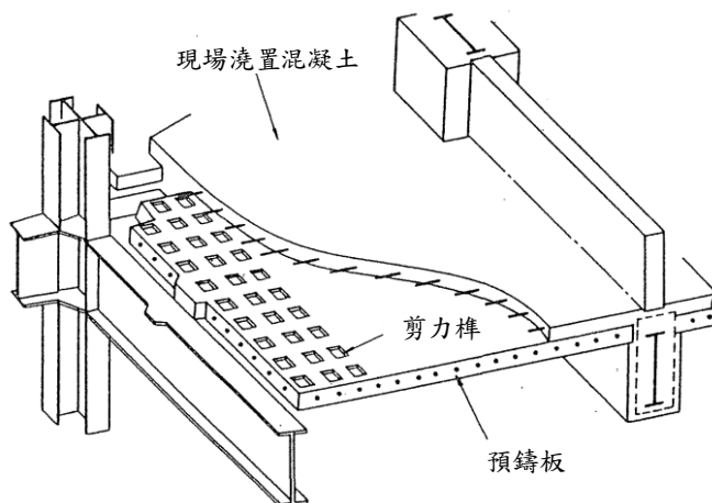
圖 R7.26 預鑄平板例 [7.5]
