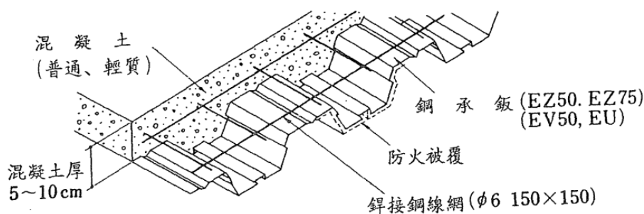
圖 R7.22 鋼承板合成樓板例(單位：mm) [7.5]
