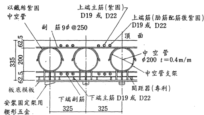
圖 R7.21 中空樓板斷面例(單位：mm) [7.5]
