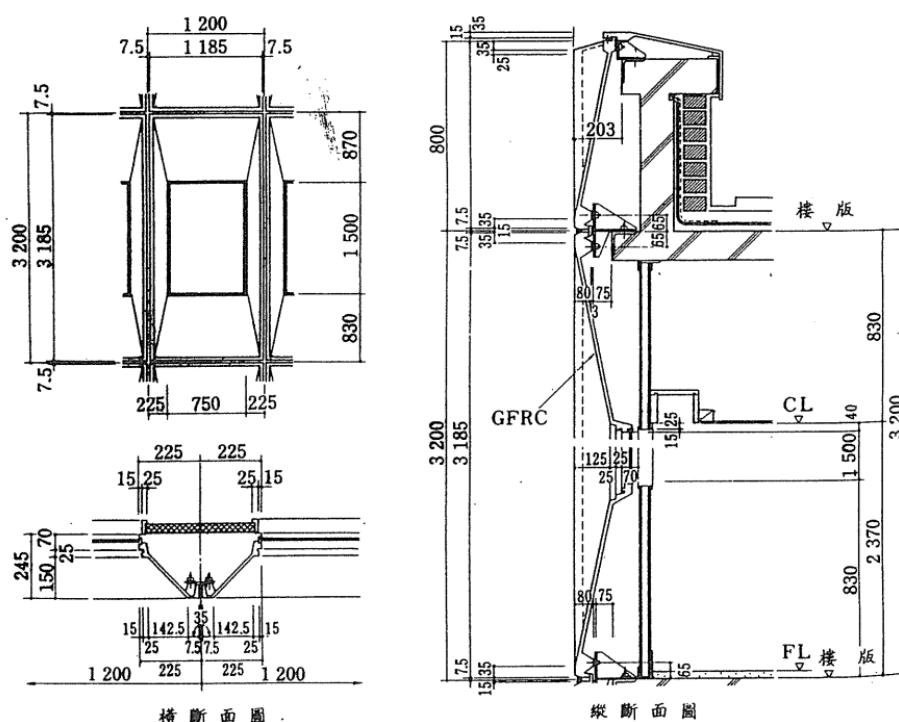
圖 R7.37 GFRC 帷幕牆圖例(單位：mm) [7.5]
