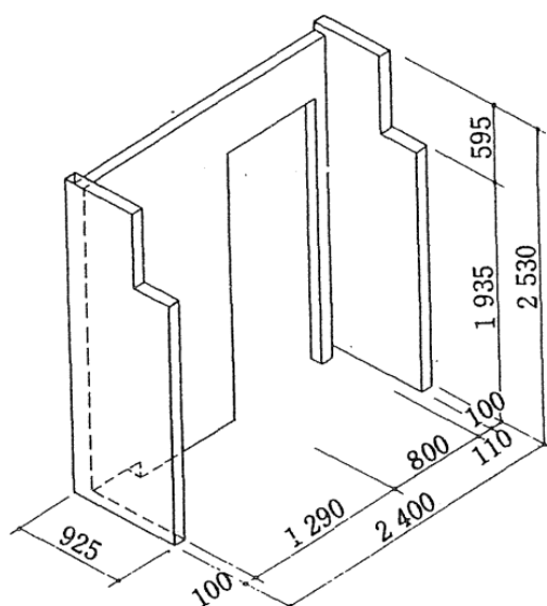
圖 R7.34 預鑄立體牆圖例(單位：mm) [7.5]
