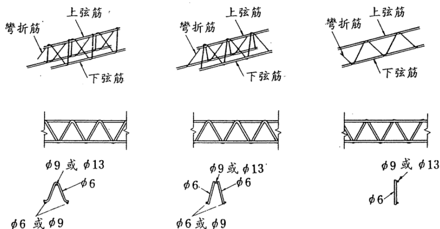
圖 R7.25 KT 筋配筋例 [7.5]
