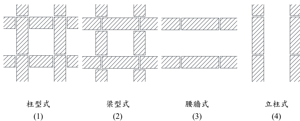
圖 R7.32 柱型、梁型組合圖例 [7.5]
