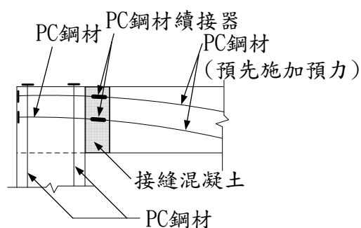
圖 R7.20 減小二次應力之接合法例 [7.5]
