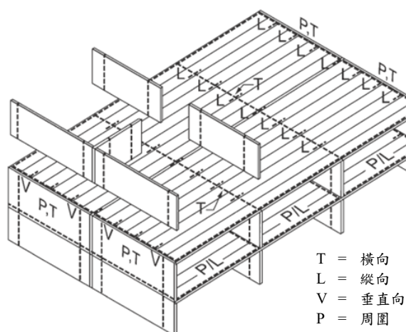
圖 R8.1 PCI 提供承重牆結構之典型整體性連接筋(integrity tie)配置 [8.2]
