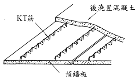
圖 R7.24 預鑄 KT 板例 [7.5]
