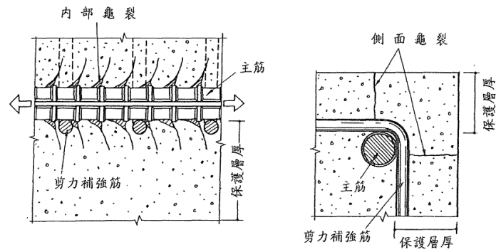
圖 R7.14 握裹破壞之機制示意圖 [7.5]
