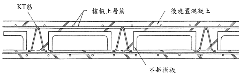
圖 R7.27 中空合成樓板例 [7.5]
