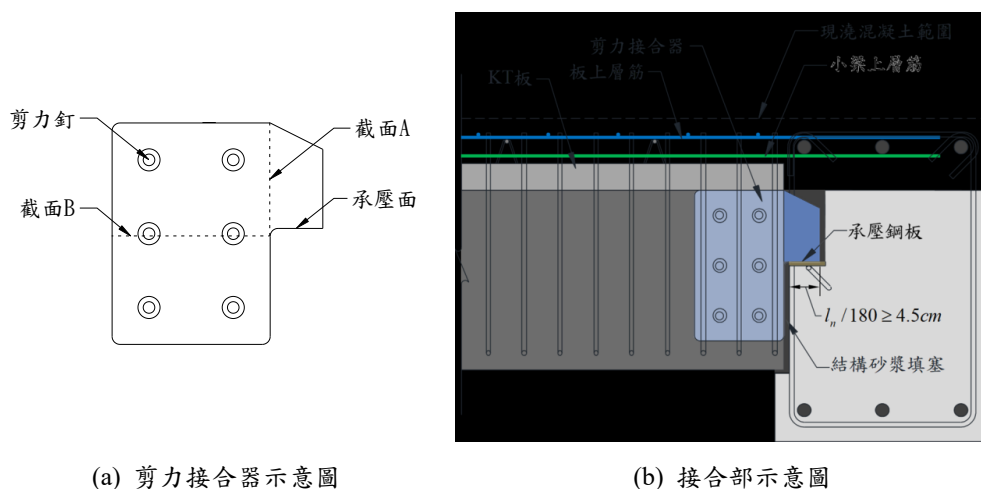
圖 R8.3 剪力接合器與接合部
