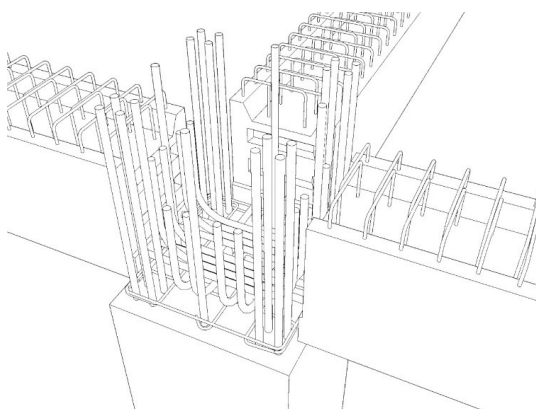
圖 R7.5 A 型工法邊柱接頭示意圖
