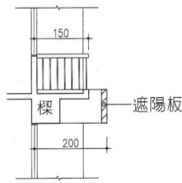
陽台面積計算 圖例 4
