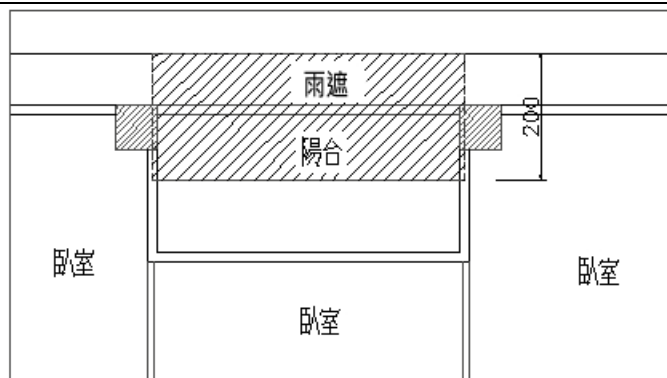
陽台面積計算 圖例 1
