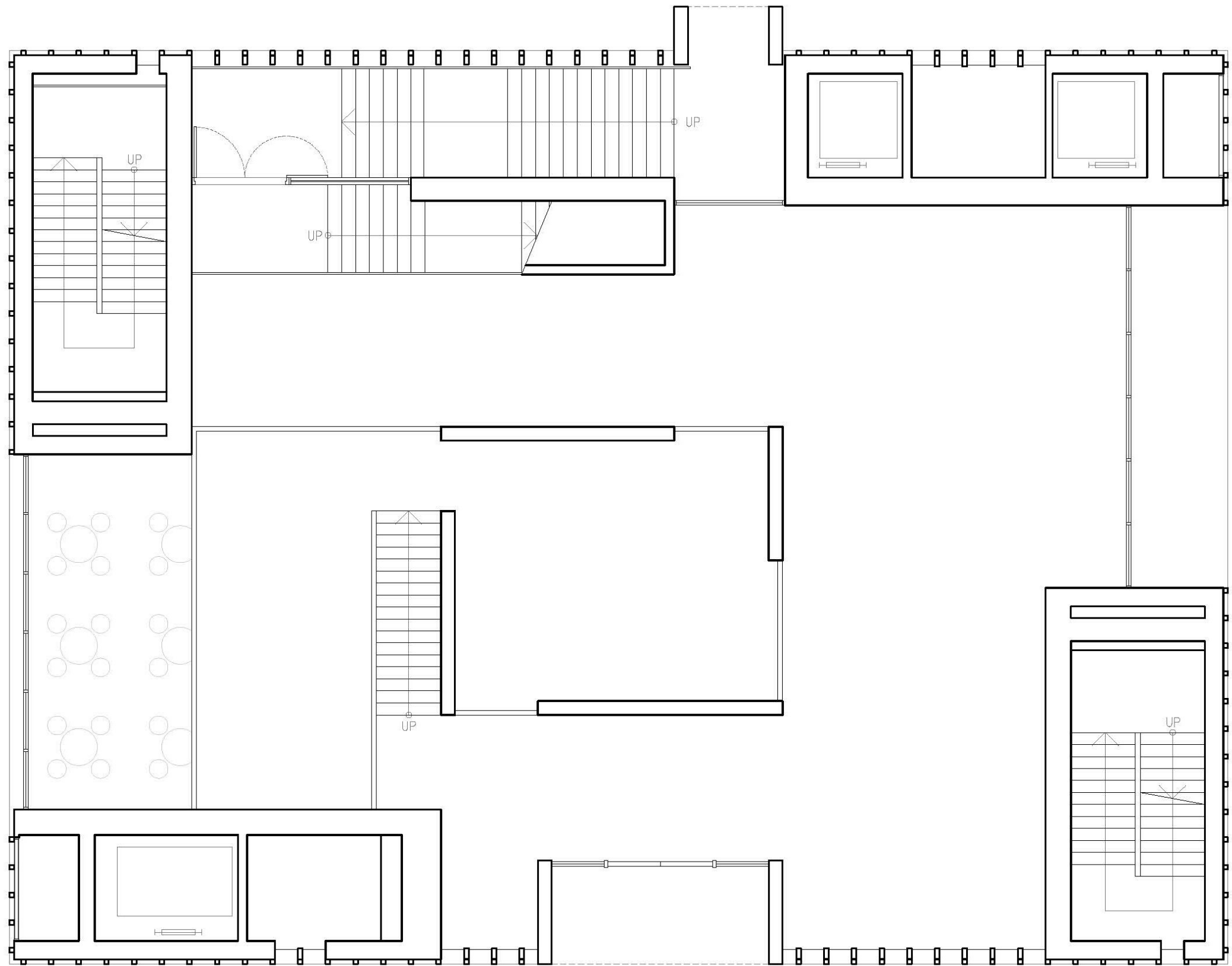
一樓夾層平面圖
