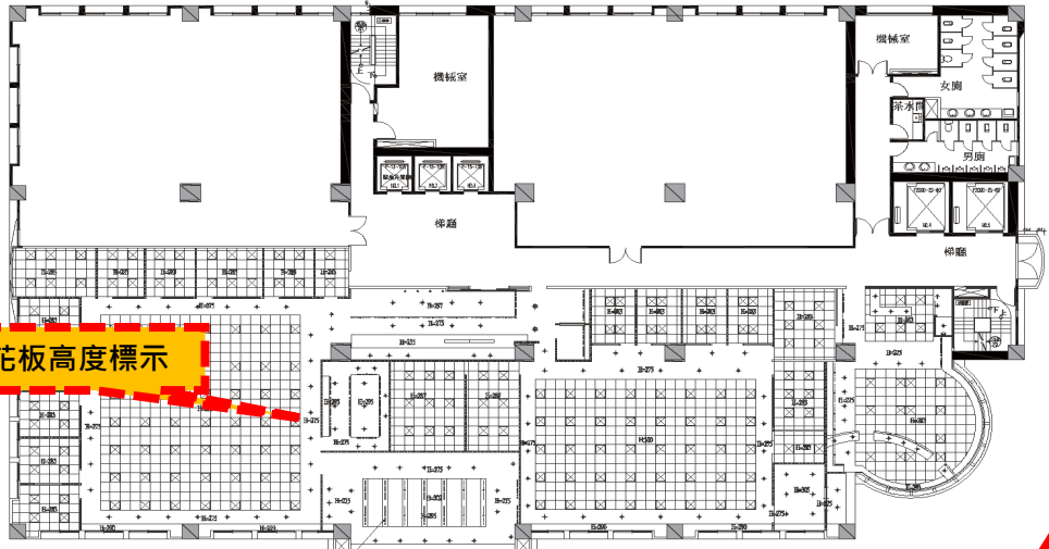
九層天花板反射平面圖S:1/100
