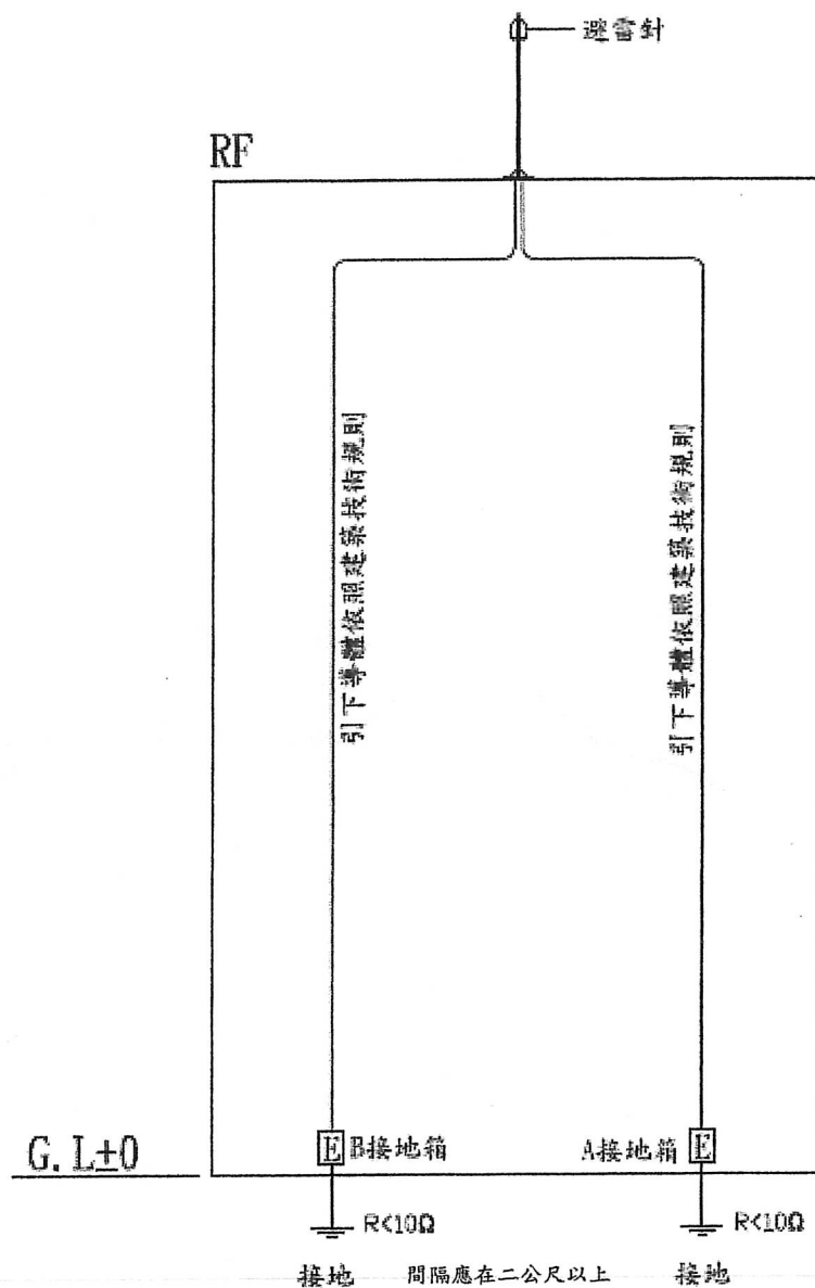
避雷系統架構圖含說明
