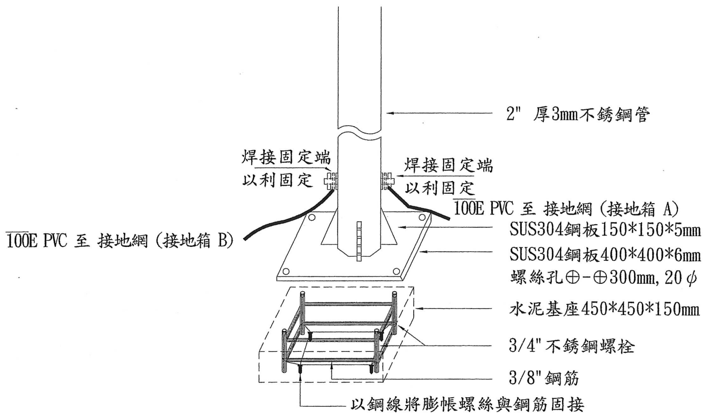
支撐架及底座圖
