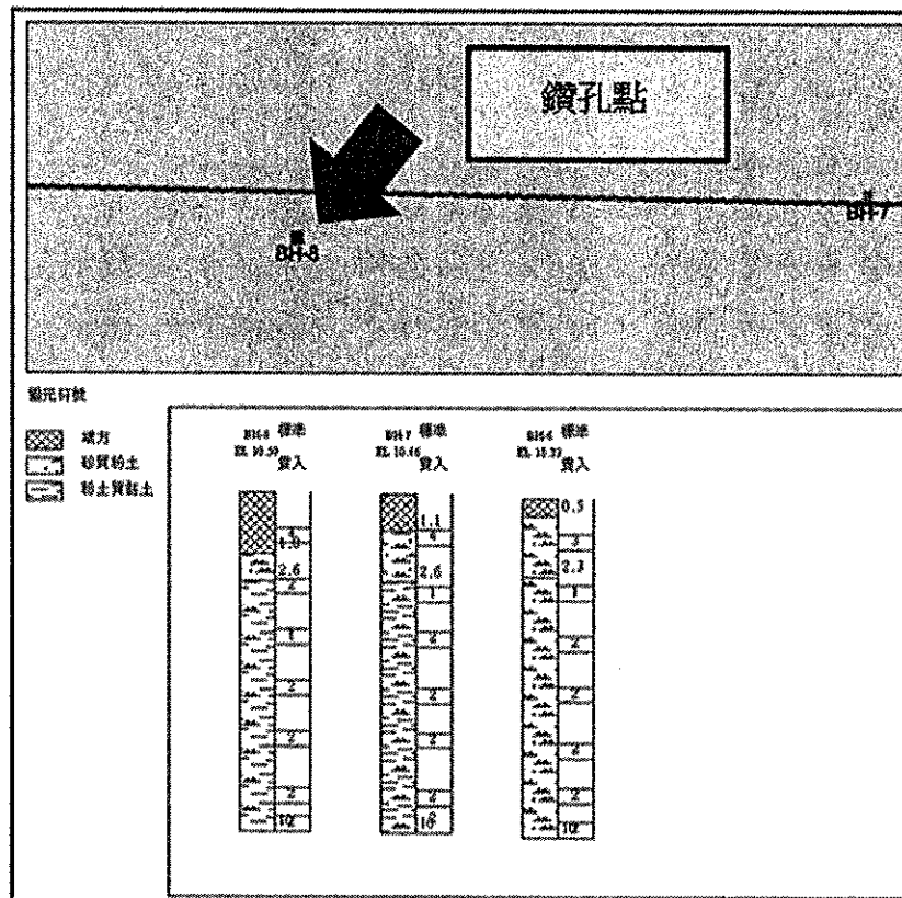
圖 6-1、工程地質探勘資料
