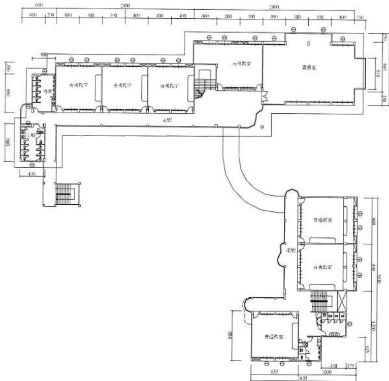
二層平面圖
