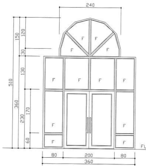
SDo 360×510 不鏽鋼落地門 五金配件齊全 裝配 10mm膠合安全玻璃
