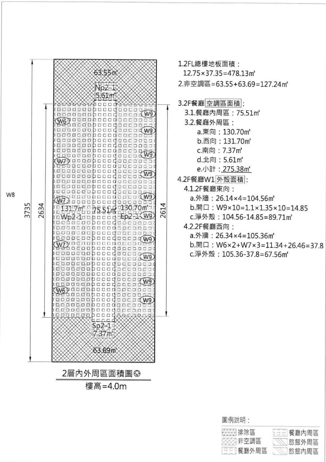
附圖 12 Envload 節能計算說明圖 4-2
