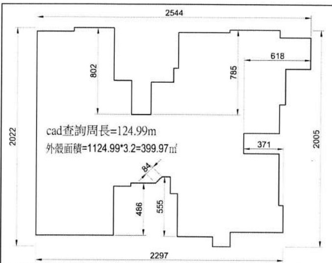
二層外殼面積計算圖
