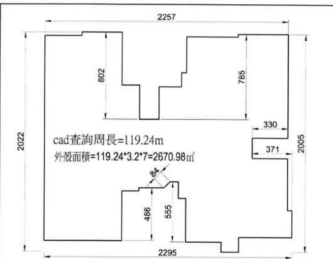
三~九層外殼面積計算圖
