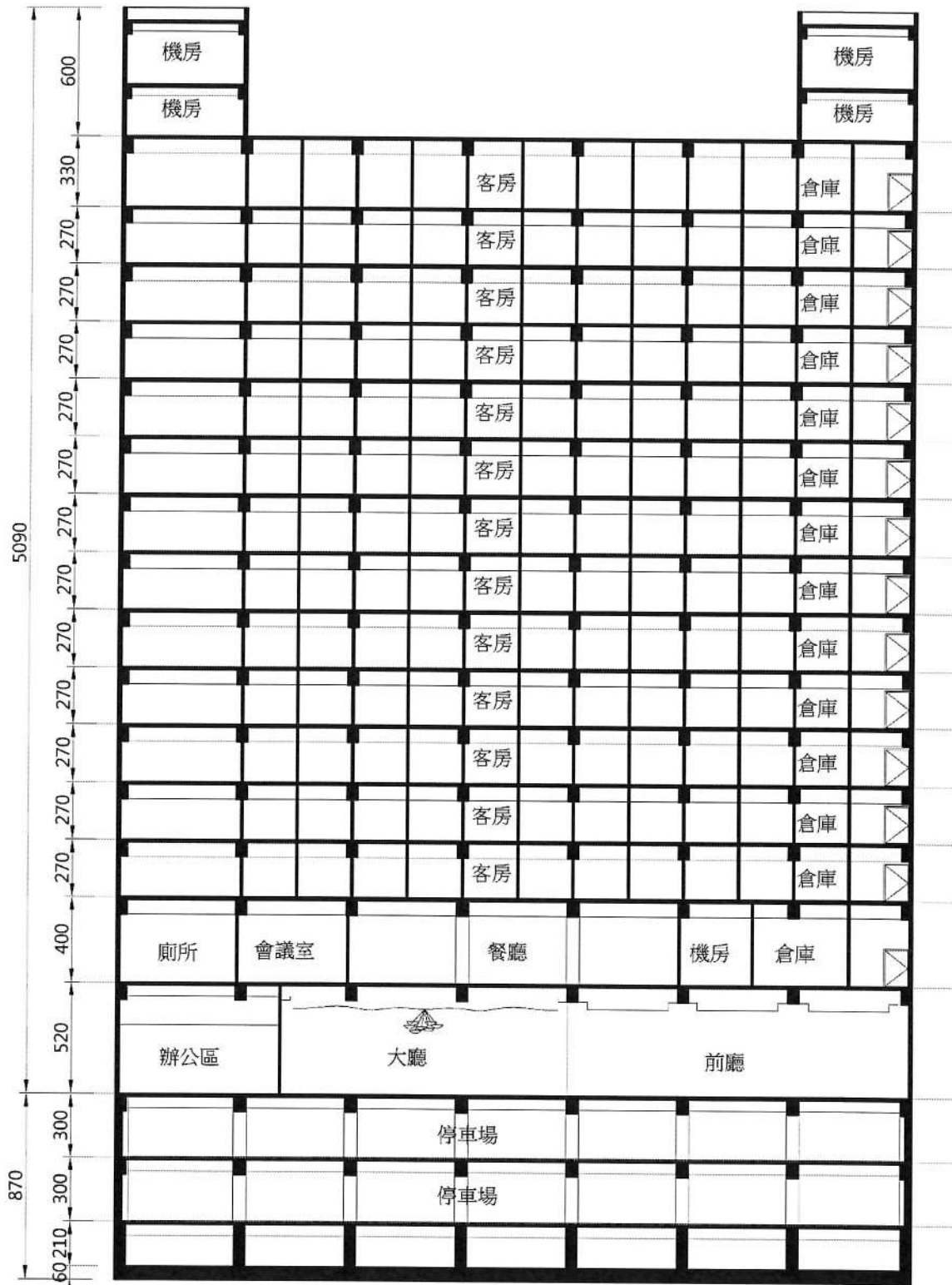
附圖 8 長向剖面圖
