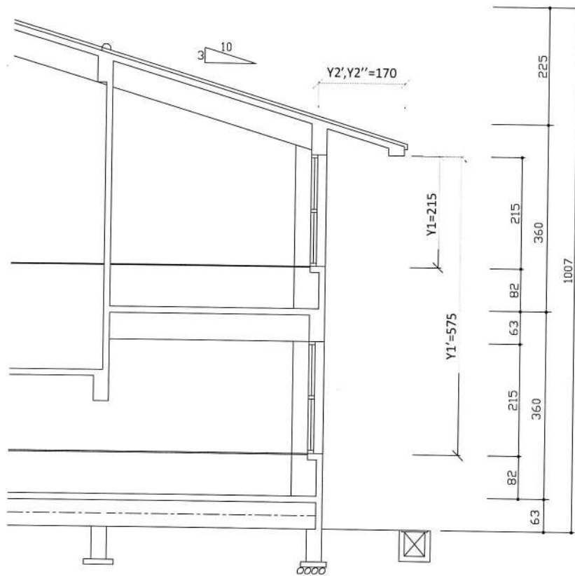
牆面剖面圖
