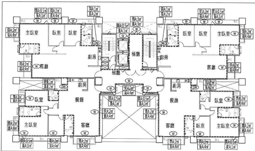
圖 1 某住宅平面「自然通風檢討面積」示意圖
