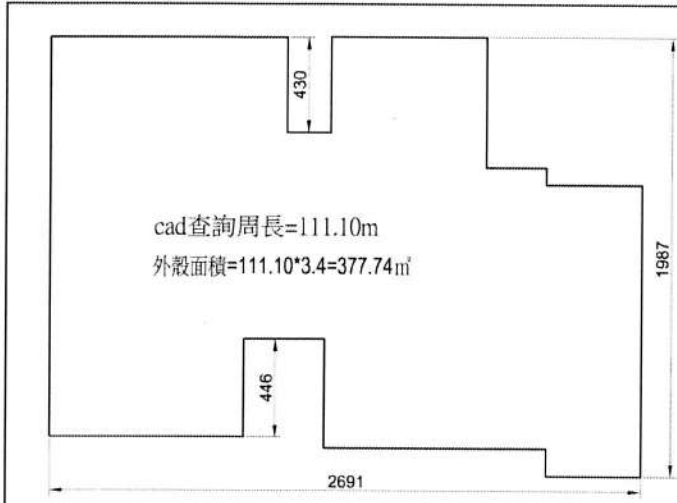
一層外殼面積計算圖
