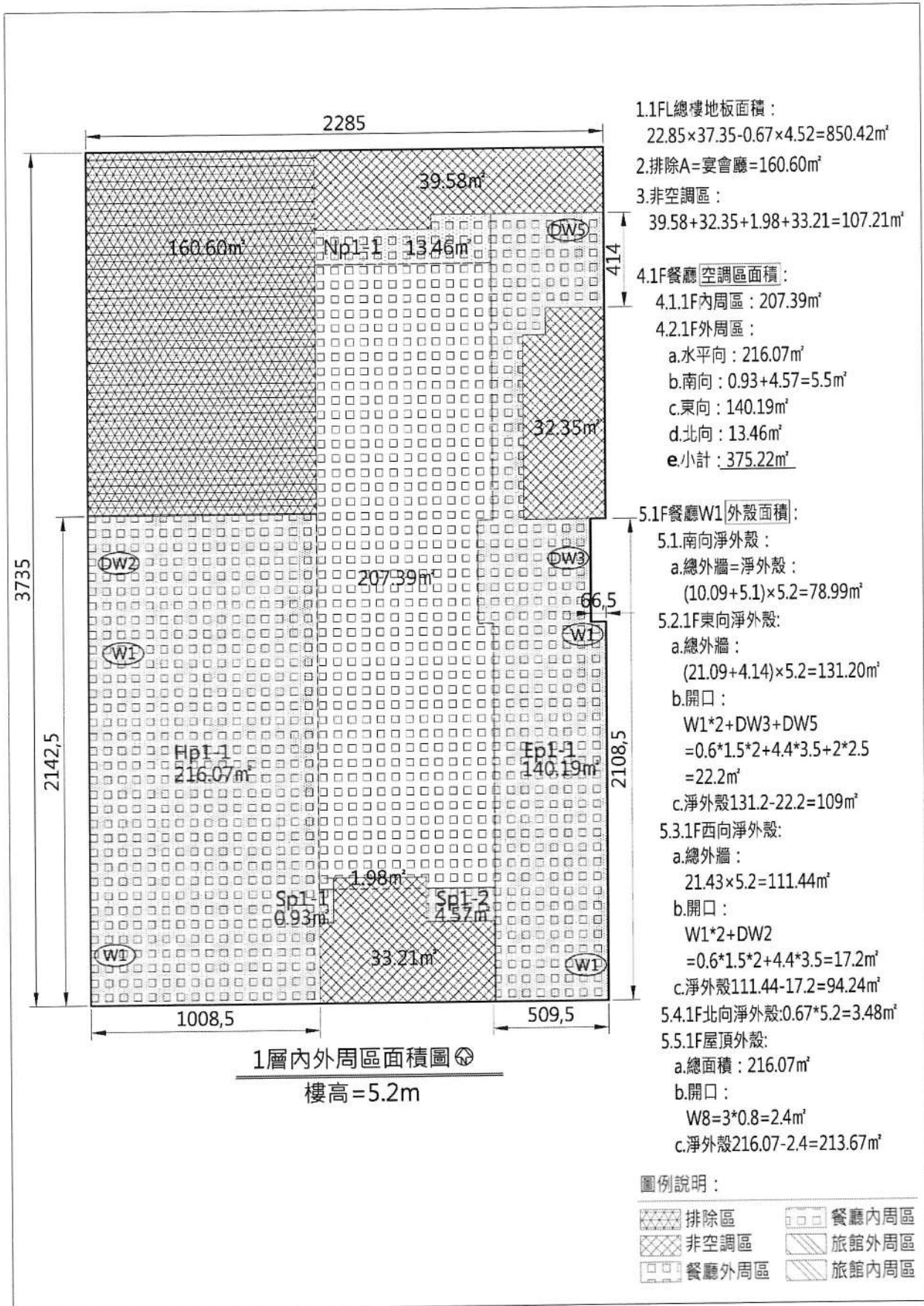
附圖 11 Envload 節能計算說明圖 4-1
