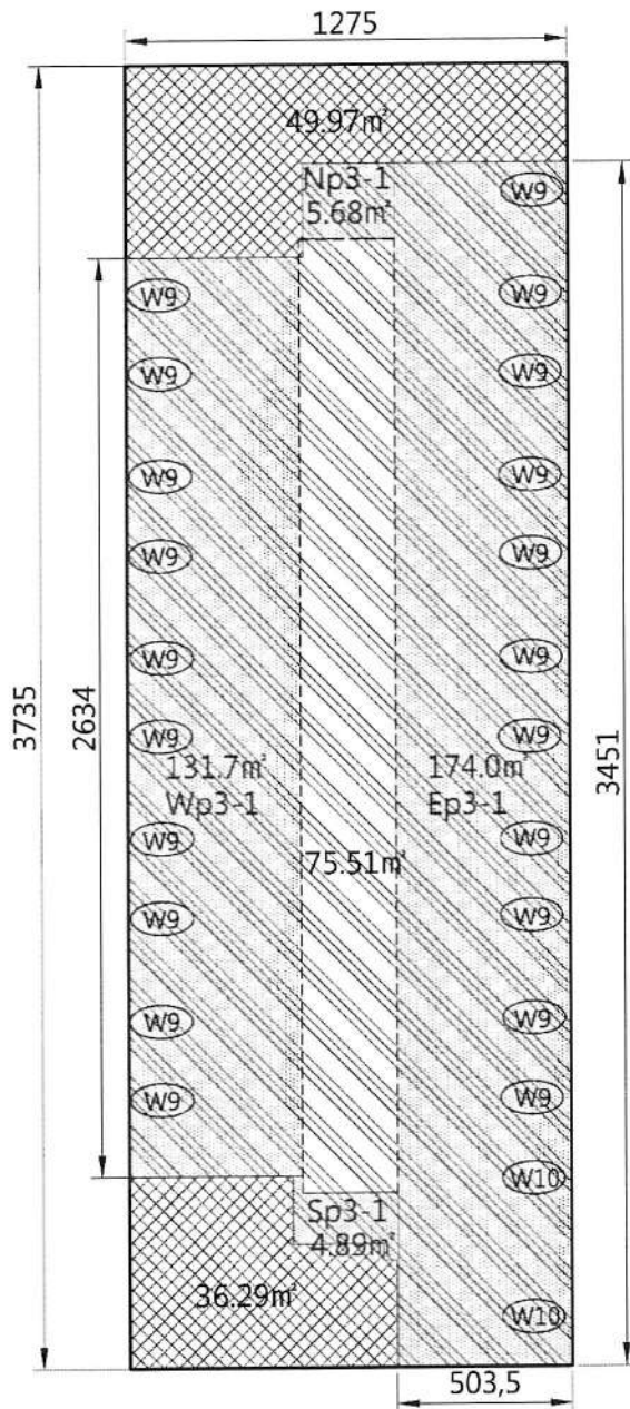
3-14層內外周區面積圖
