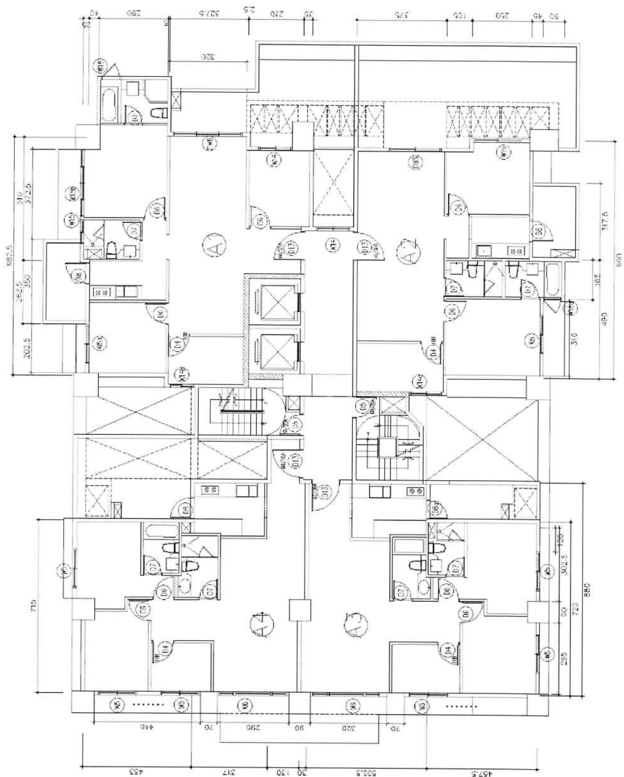
附圖 16 2F平面圖
