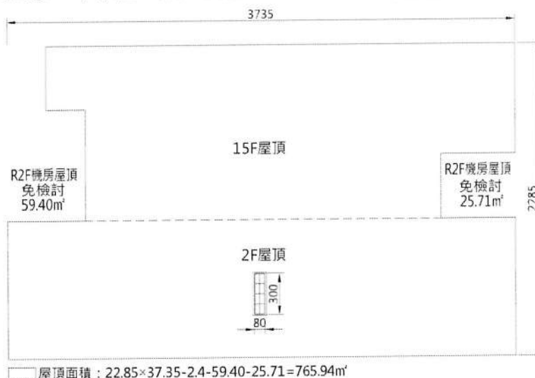
附圖 9 屋頂構造面積計算檢討圖
