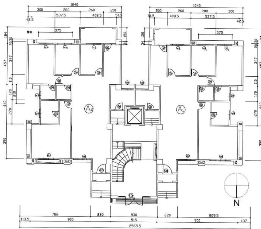
1F 平面
