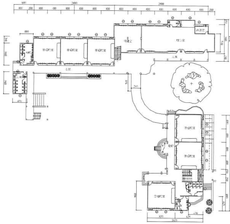
一層平面圖
