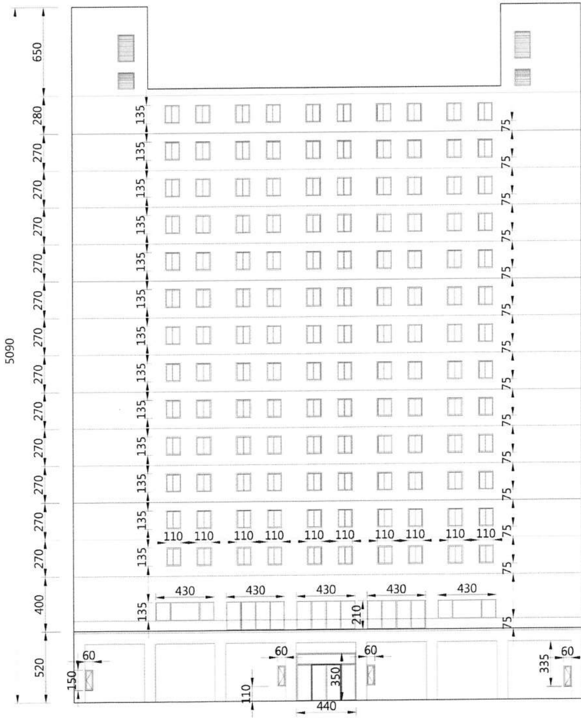
附圖 4 西向立面圖
