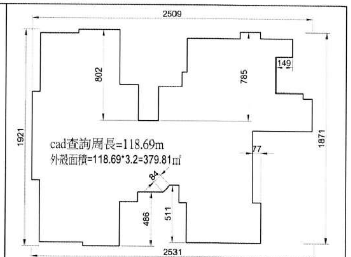
十層外殼面積計算圖
