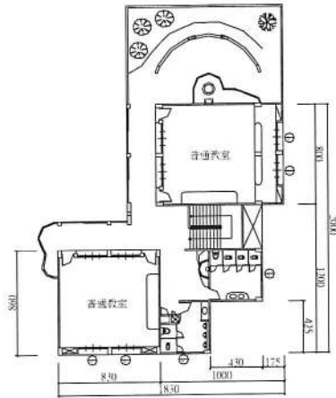
三層平面圖
