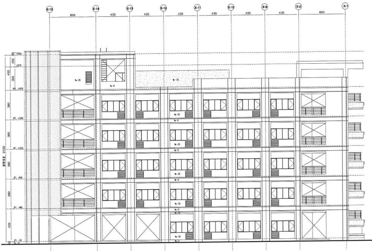
北向立面圖
