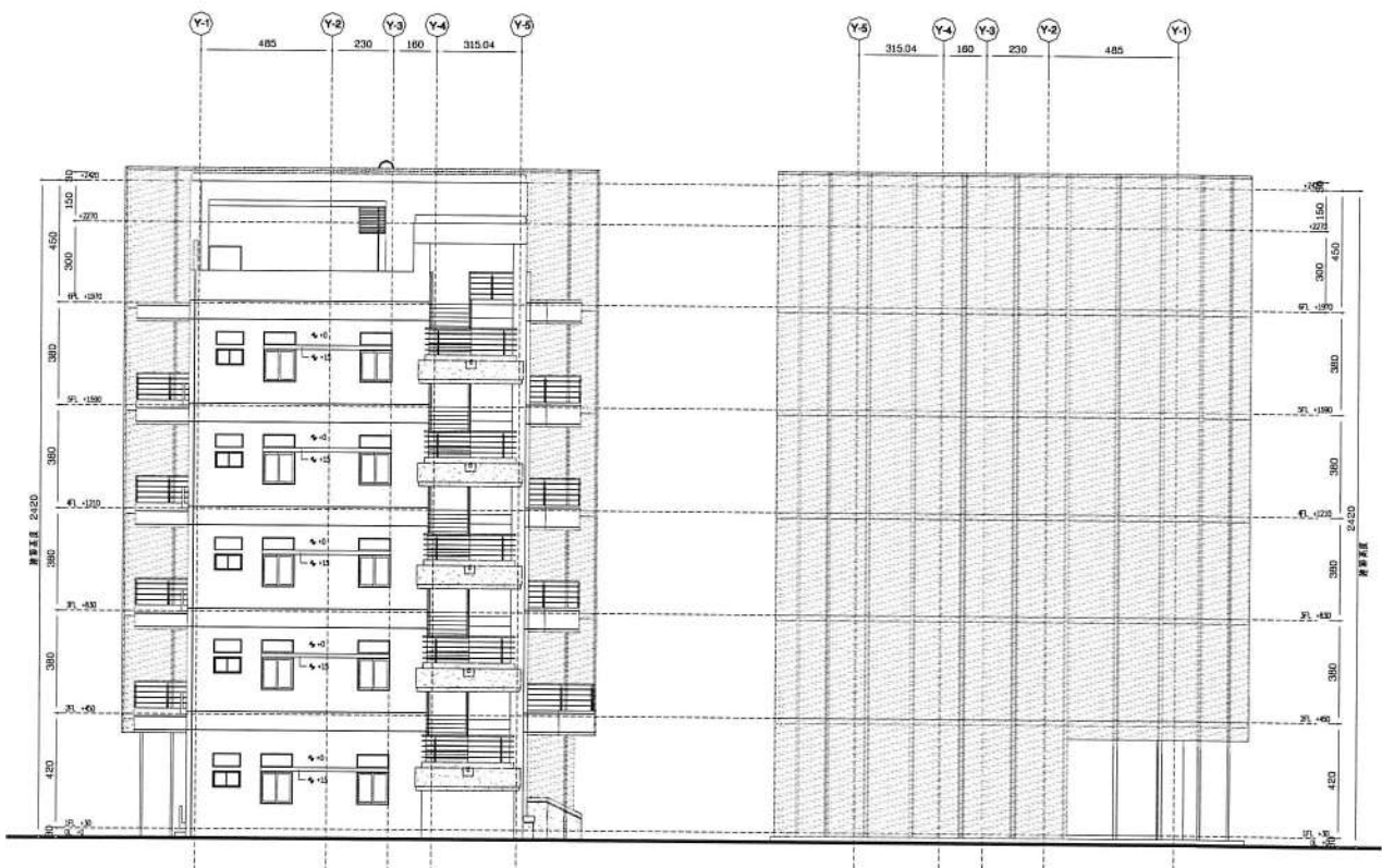
西向立面圖
