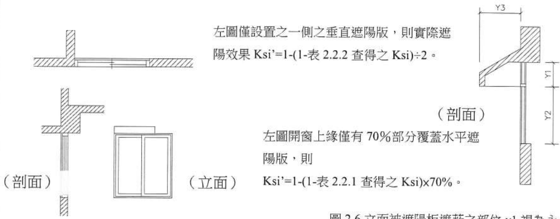
圖 2.5 局部遮陽之 K_{si}' 修正計算
