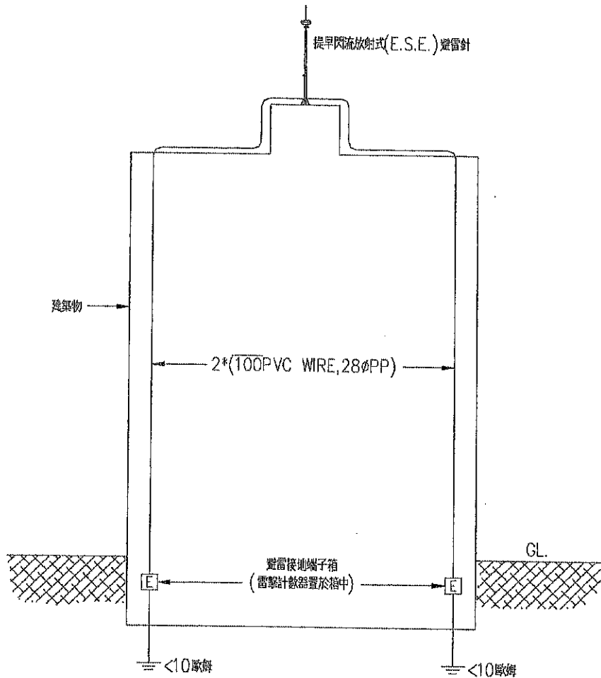
放電式避雷針裝置架構圖（一）
