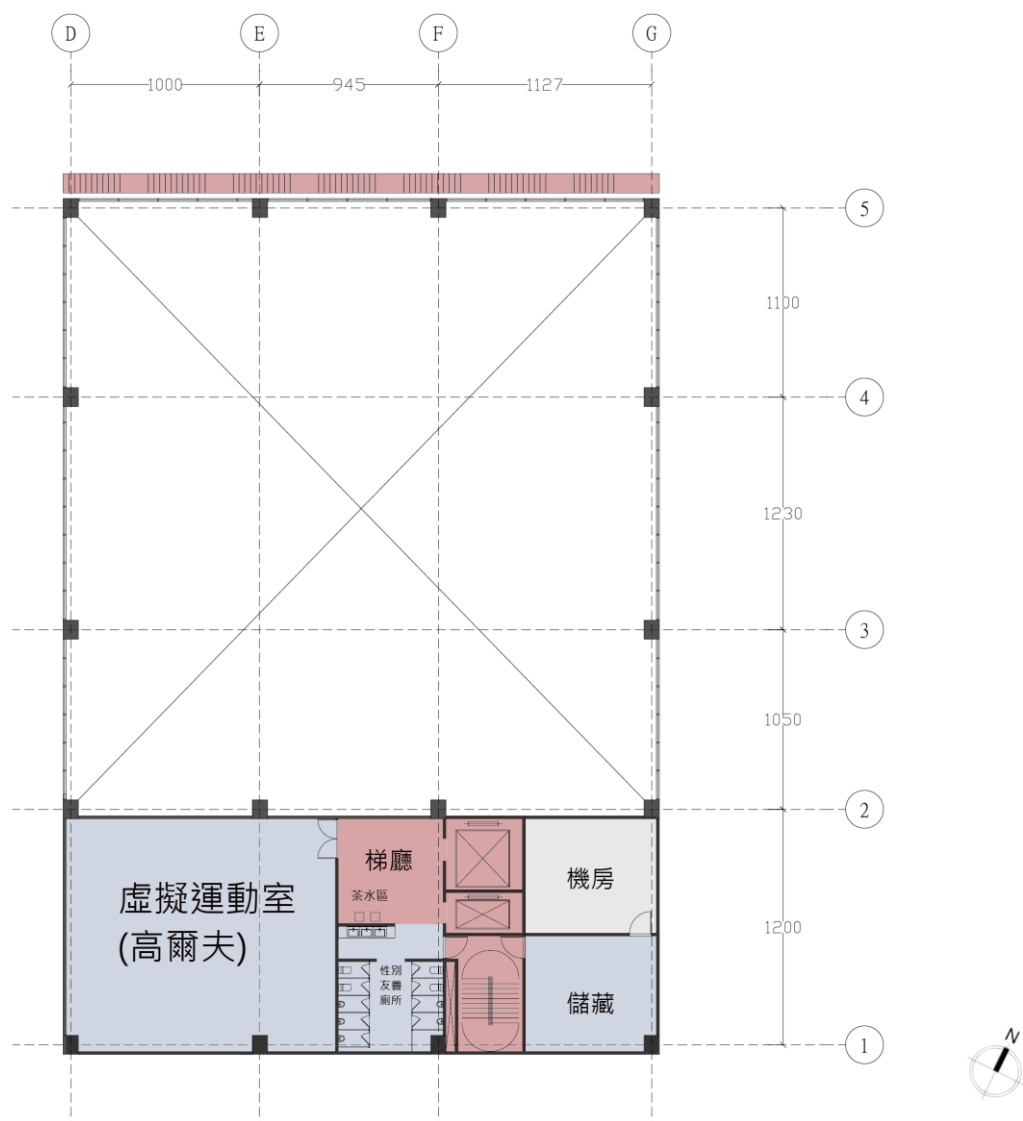
圖 12 四樓平面圖
