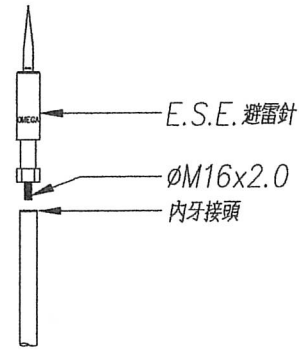
避雷針連接固定架
