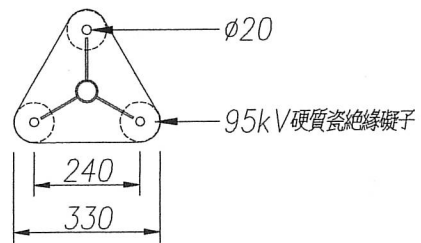
固定架底座
