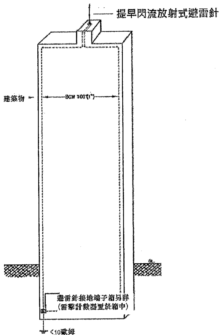
閃流放射式避電針裝置配線圖
