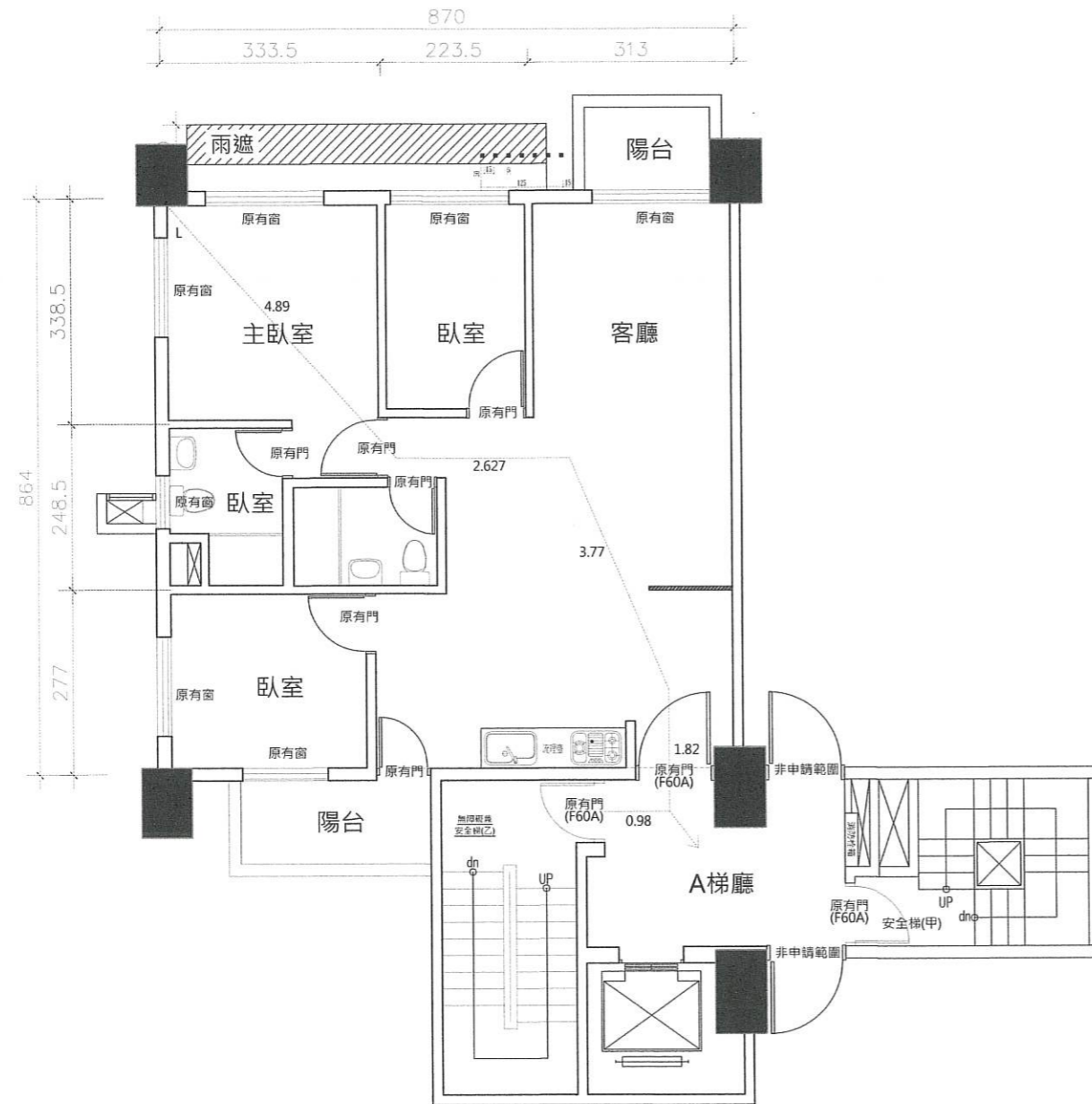
八樓裝修竣工平面圖 S : 1/100
