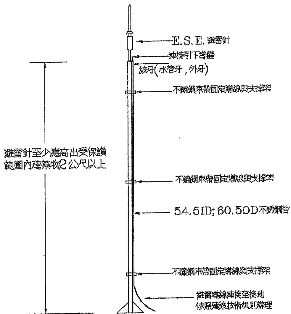
避雷針典型組立圖 不同現場狀況可能會有不同的組立方式
